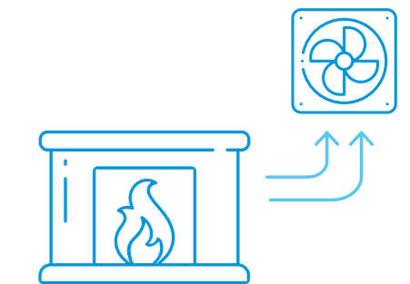
Išmatuota kambario temperatūra ≥ nustatyta temperatūra = terminė įranga išjungiama Automatinis ventiliatoriaus reguliavimas pagal ΔT
